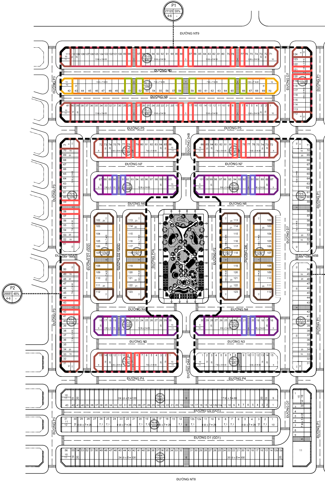
MẶT BẰNG TỔNG THỂ VỊ TRÍ LẬP BẢO CÁO NGHIÊN CỨU KHẢ THI KHU NHÀ Ở PRINCE TOWN II (MỞ RỘNG) - P1, P2, P3
