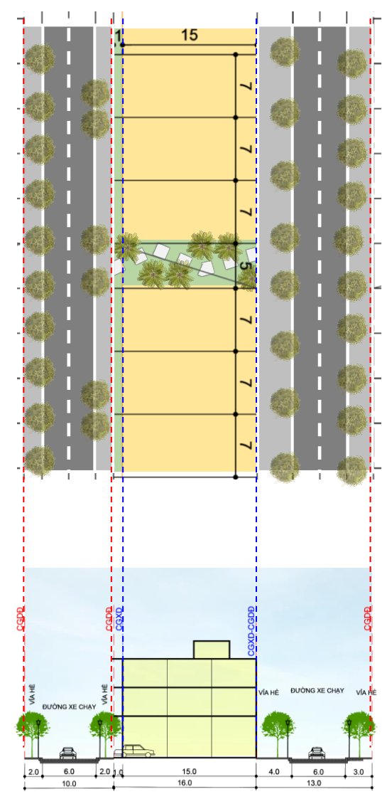
MẶT CẮT 3-3
