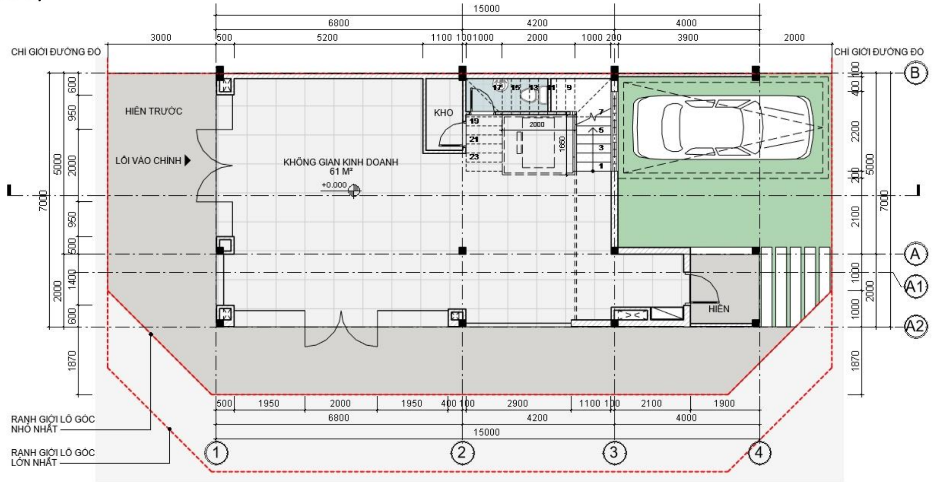
MẶT BẰNG TẦNG 1
