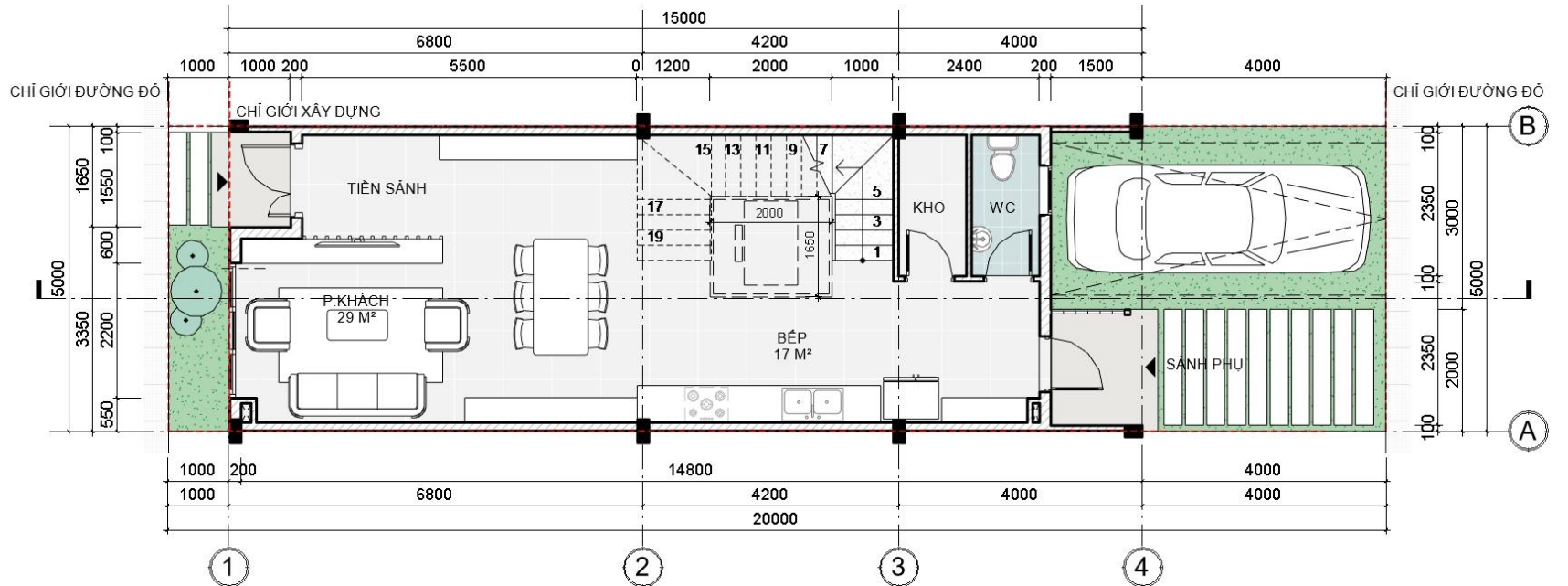
MẶT BẰNG TẦNG 1
