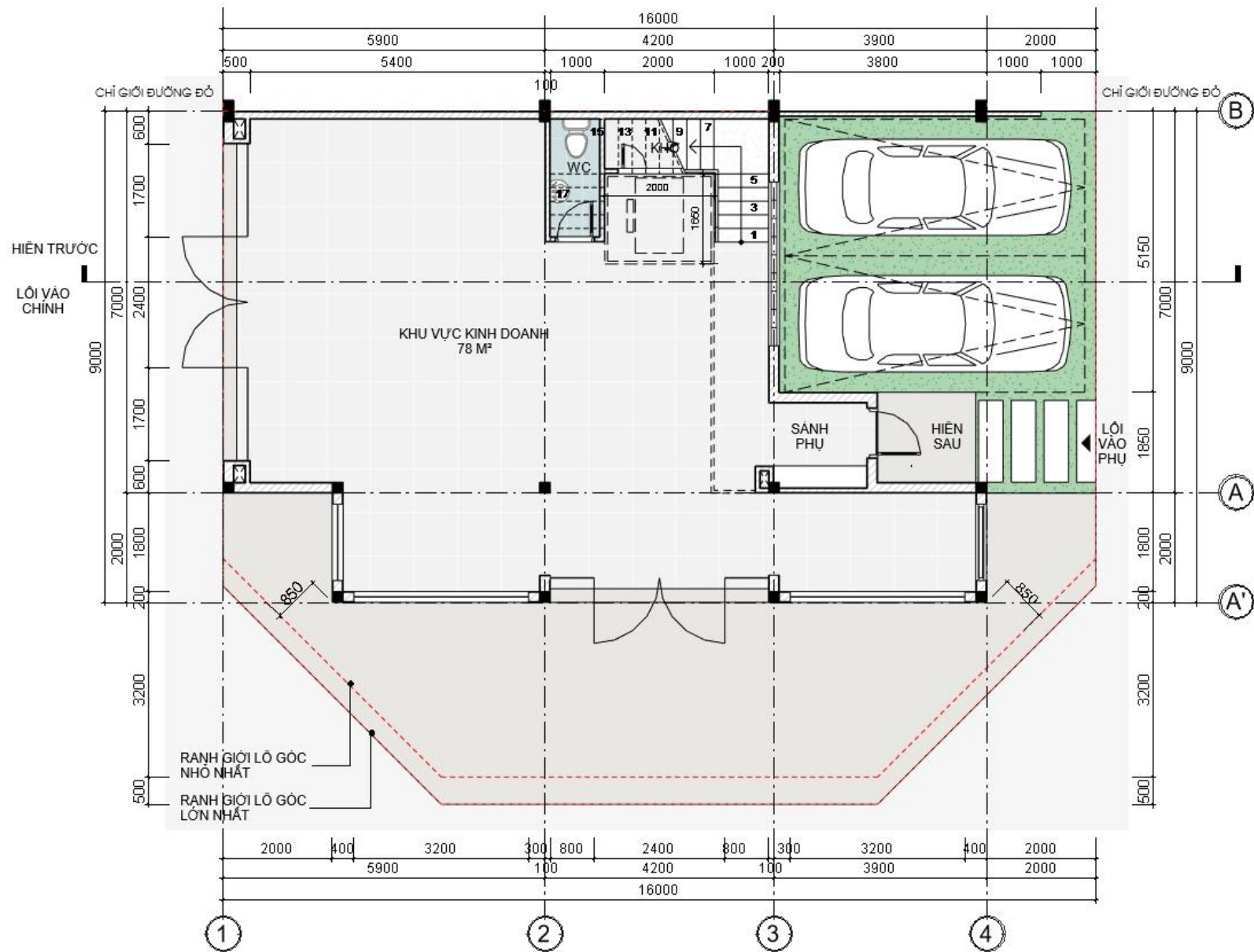
MẶT BẰNG TẦNG 1
