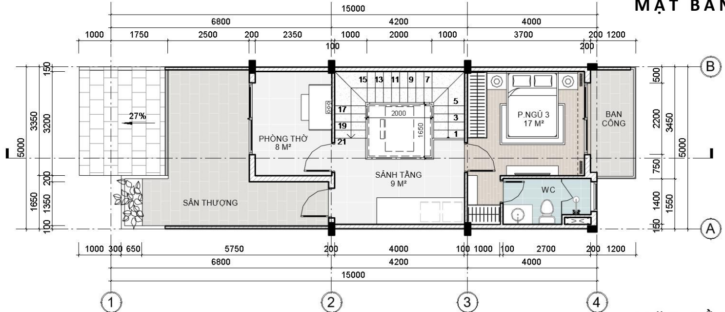
MẶT BẰNG TẦNG 4
