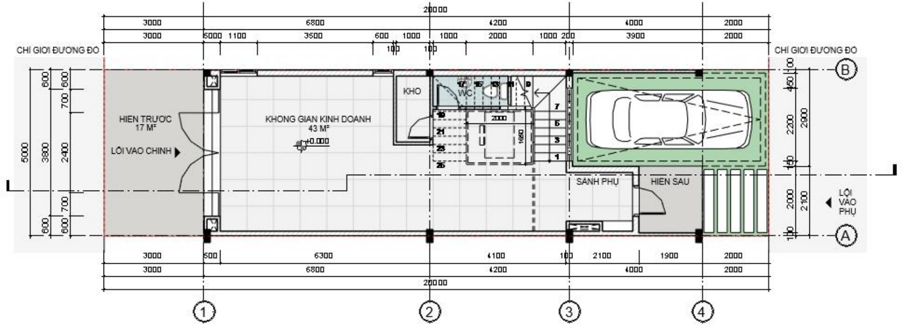
MẶT BẰNG TẦNG 1
