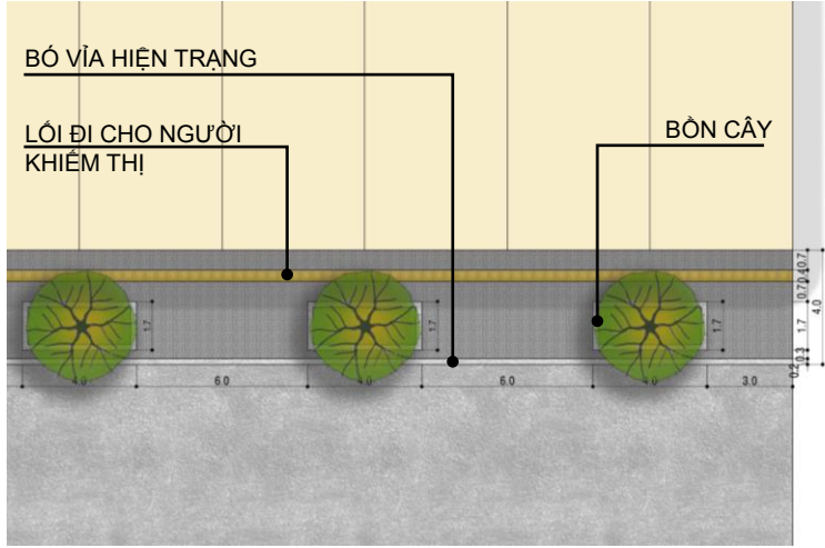
QUY CÁCH LÁT VÍA HÈ
