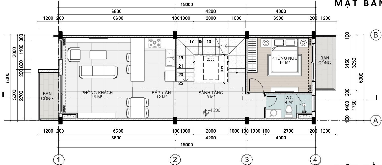
MẶT BẰNG TẦNG 2
