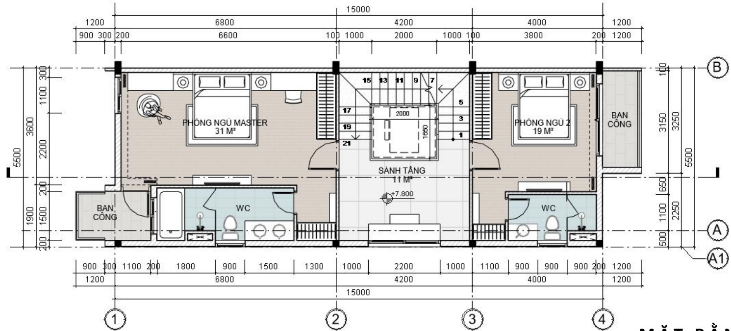
MẶT BẰNG TẦNG 3
