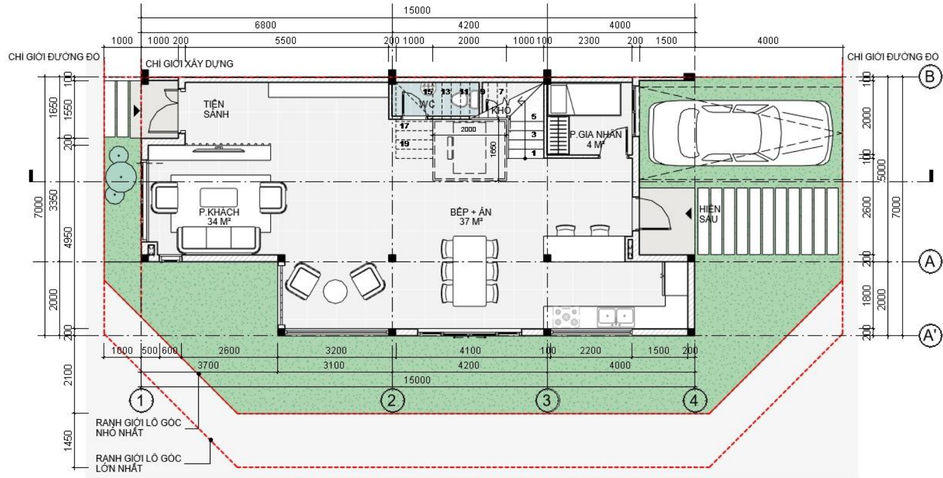
MẶT BẰNG TẦNG 1
