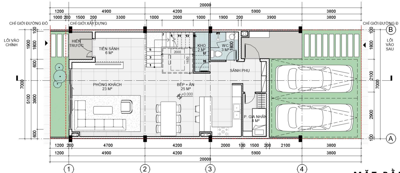
MẶT BẰNG TẦNG 1
