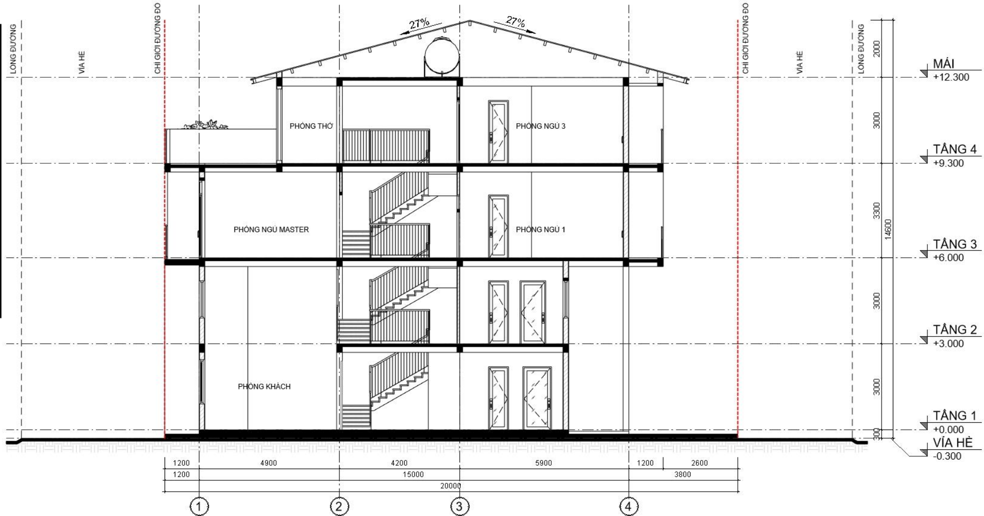
MẶT CẮT
