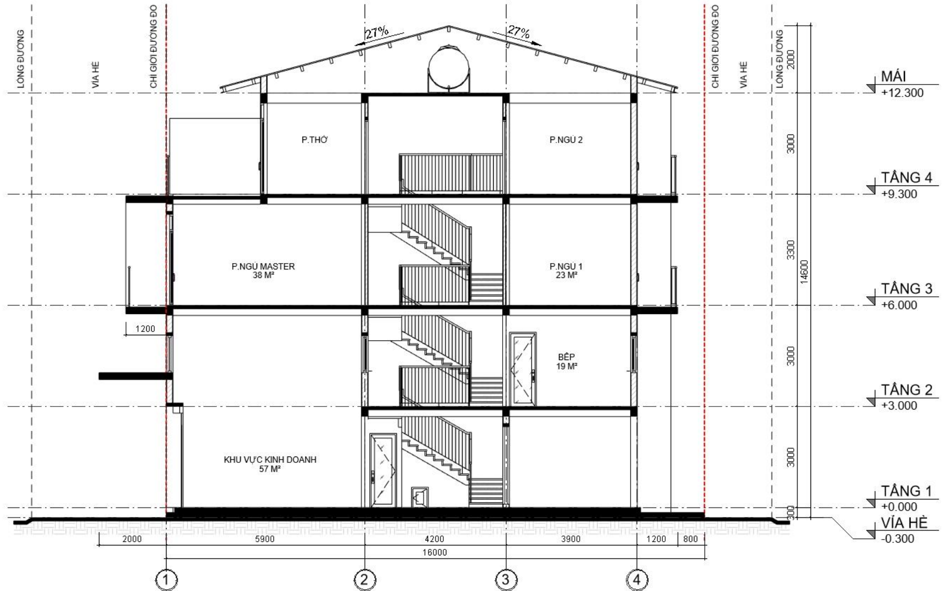
MẶT CẮT
