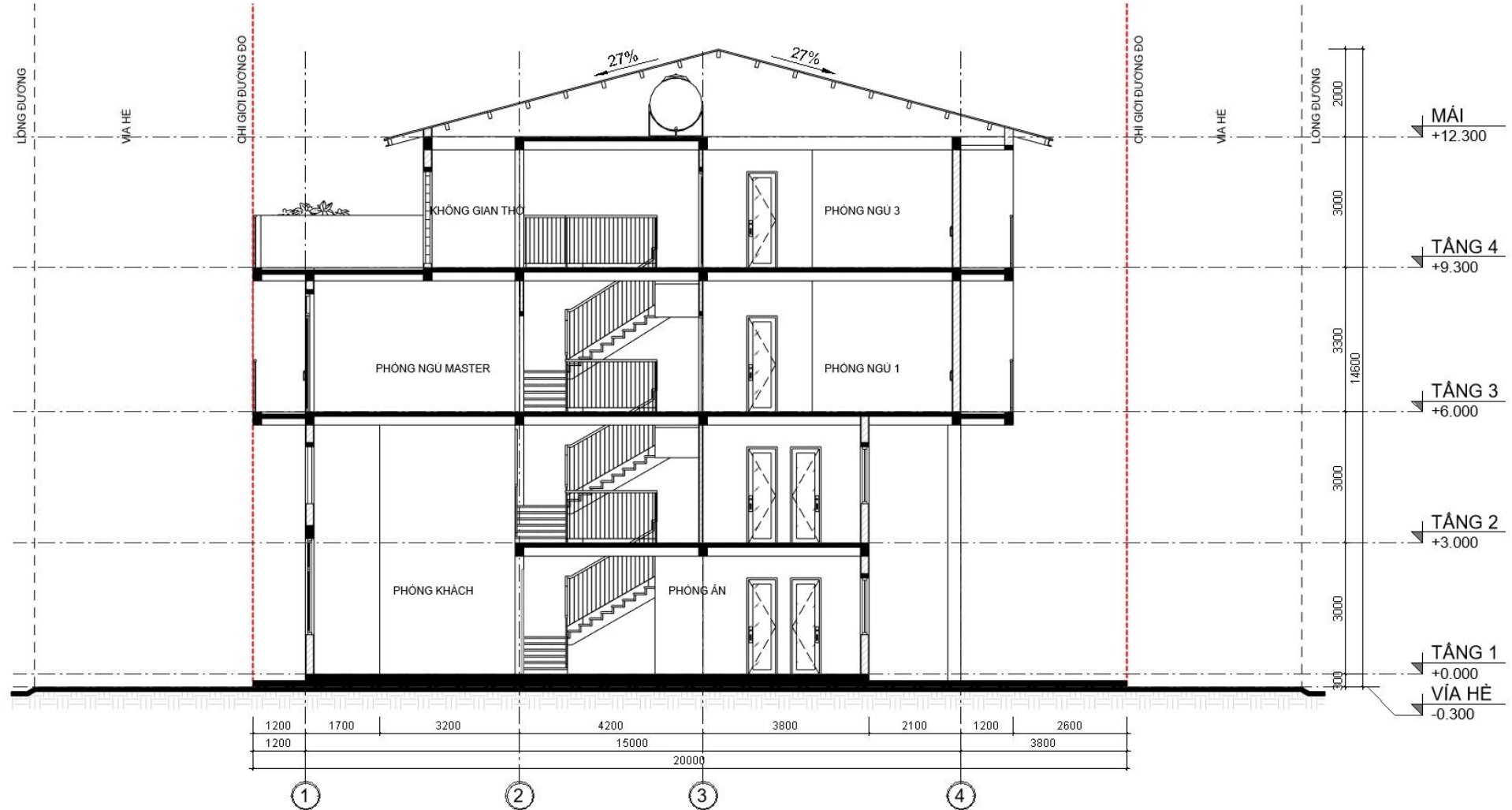
MẶT CẮT
