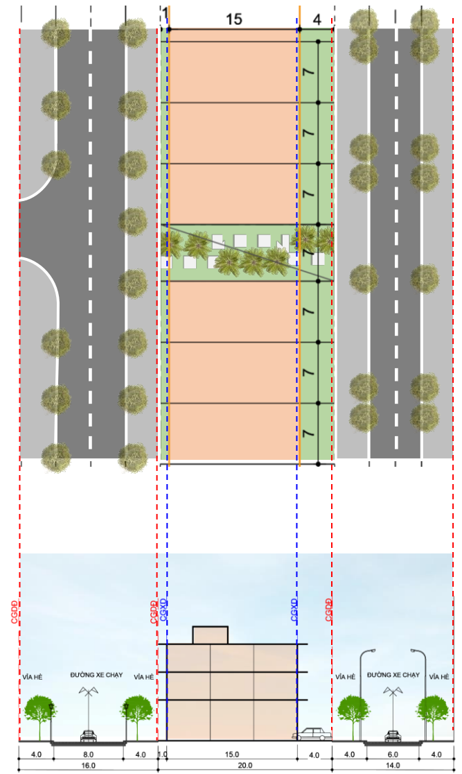
MẶT CẮT 2-2
