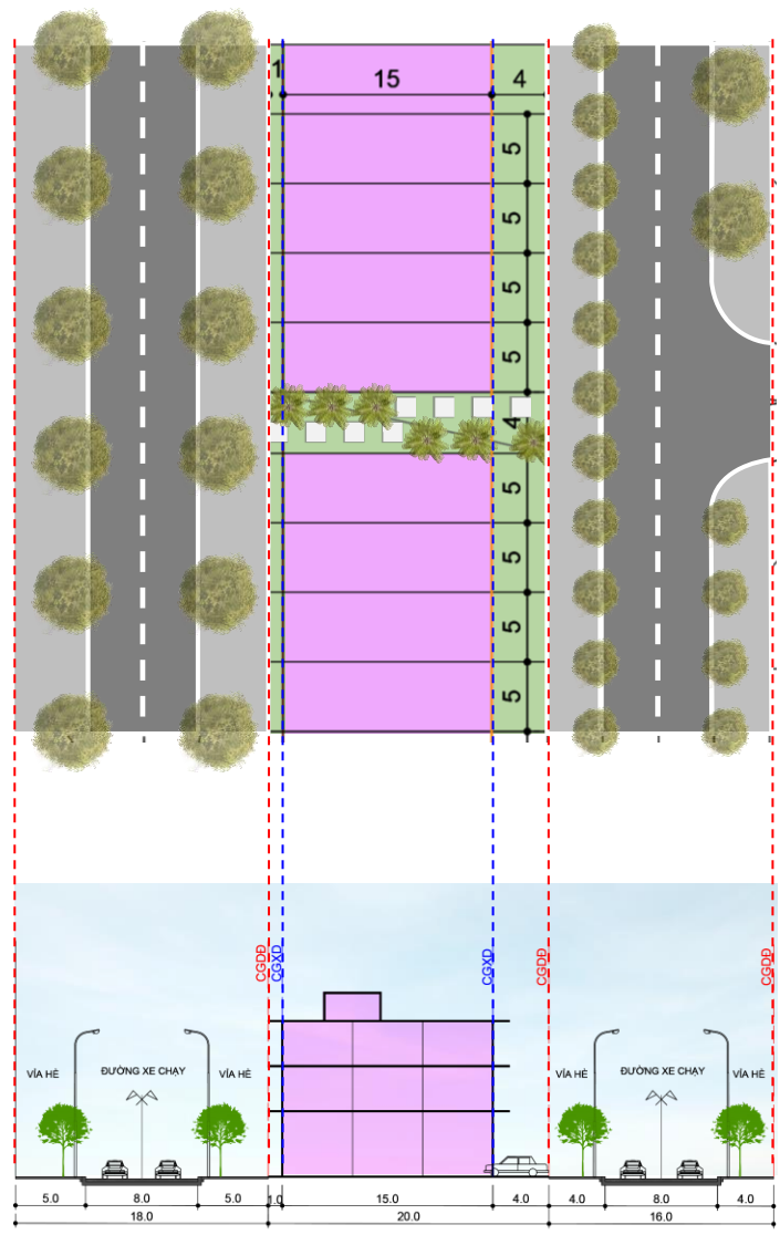
MẶT CẮT 1-1
