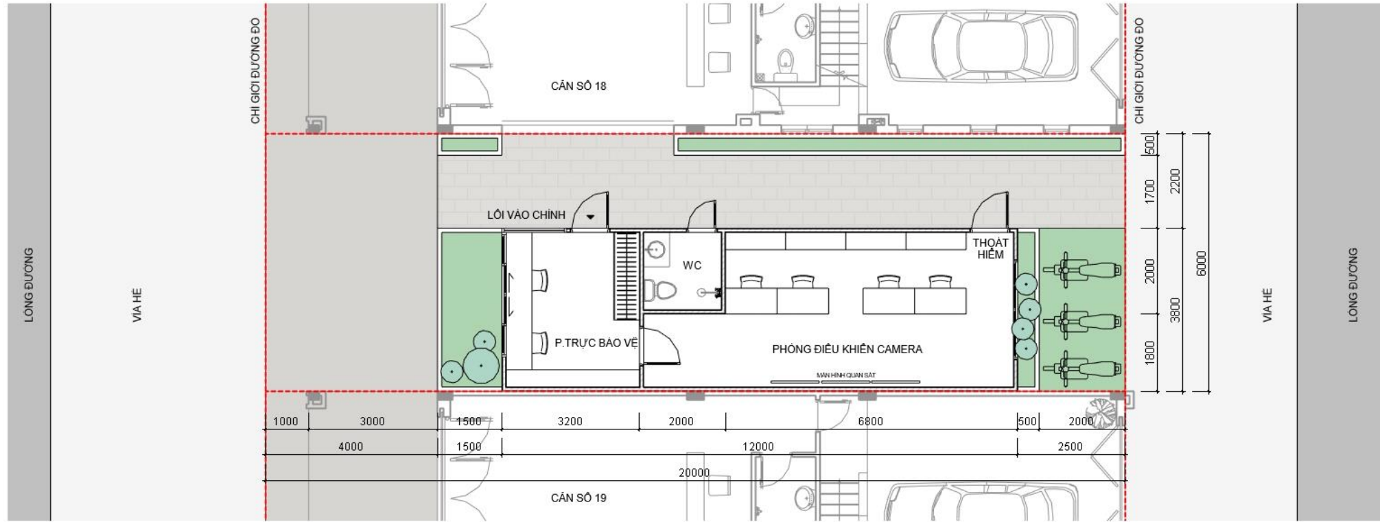
MẶT BẰNG BỐ TRÍ CHỐT KIỂM SOÁT AN NINH & PHÒNG ĐIỀU KHIỂN CAMERA
