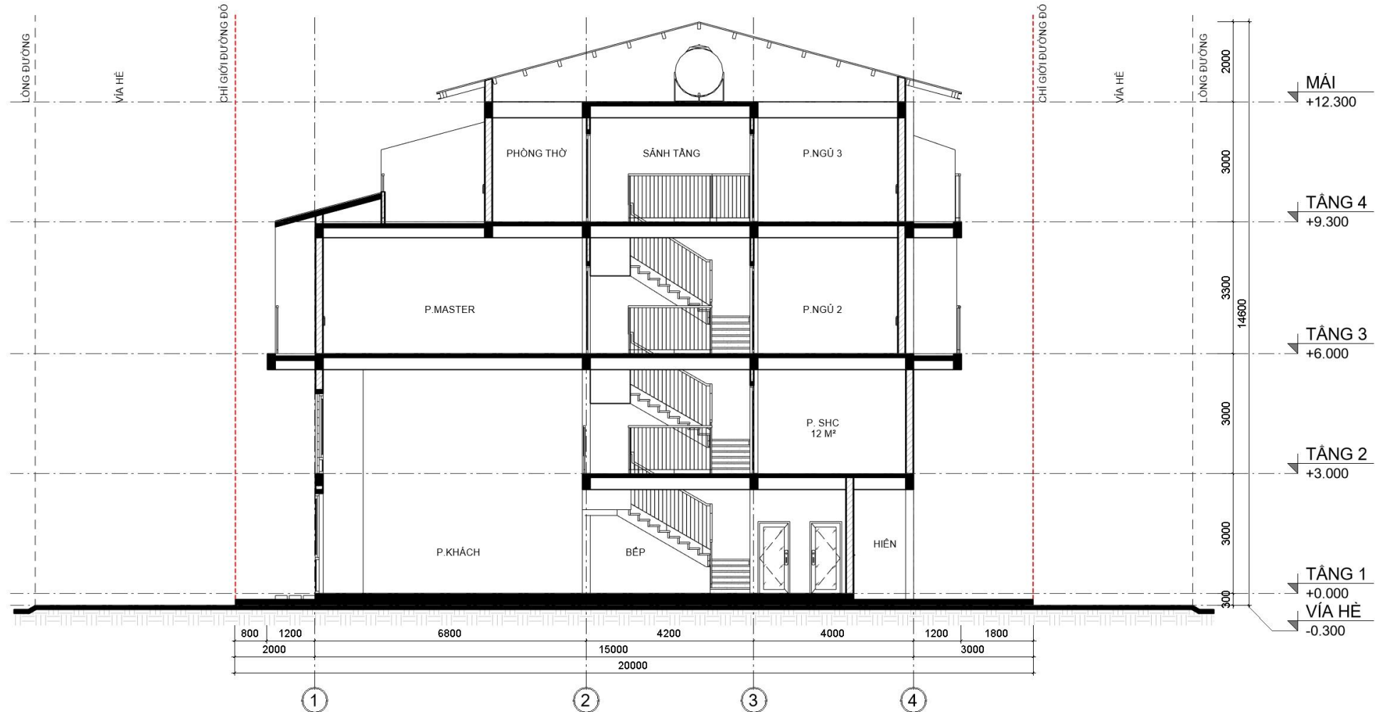
MẶT CẮT
