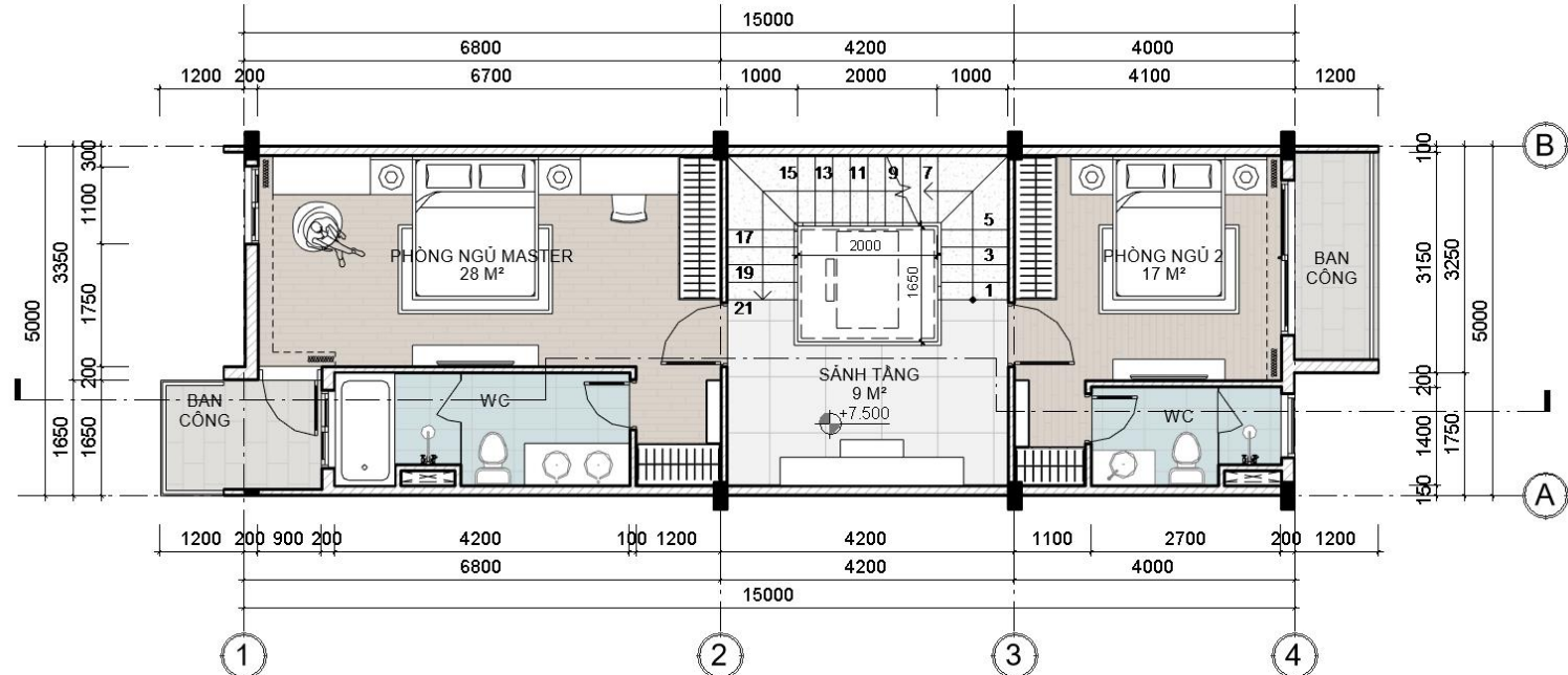
MẶT BẰNG TẦNG 3
